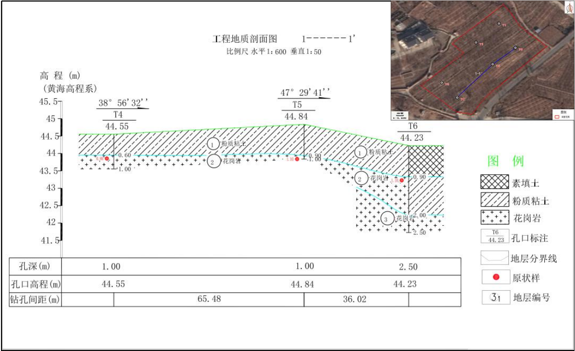
图 3.1-6 参考地块工程地质剖面图 (1-1' )
