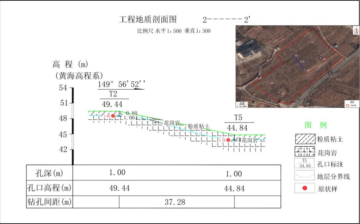
图 3.1-7 参考地块工程地质剖面图 (2-2' )
