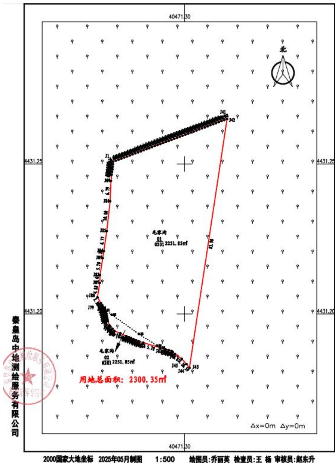
图 2.4-1 调查地块勘测定界图
