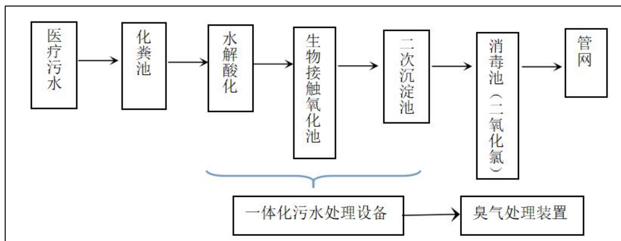
图 4.4-2 污水处理工艺
