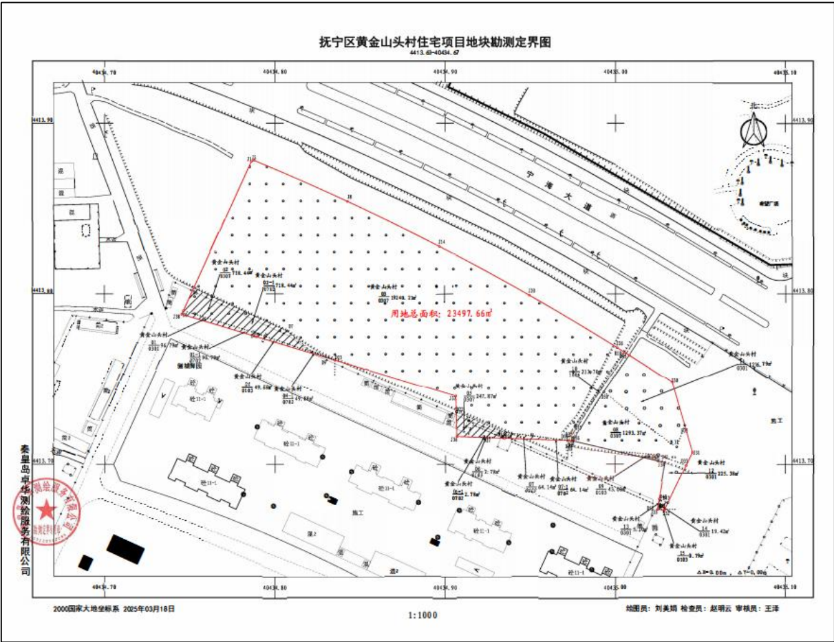
图 2.4-1 调查地块勘测定界图
