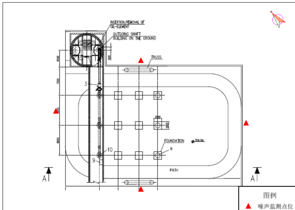
图 6.2-1 类比地面出线场噪声监测点位
