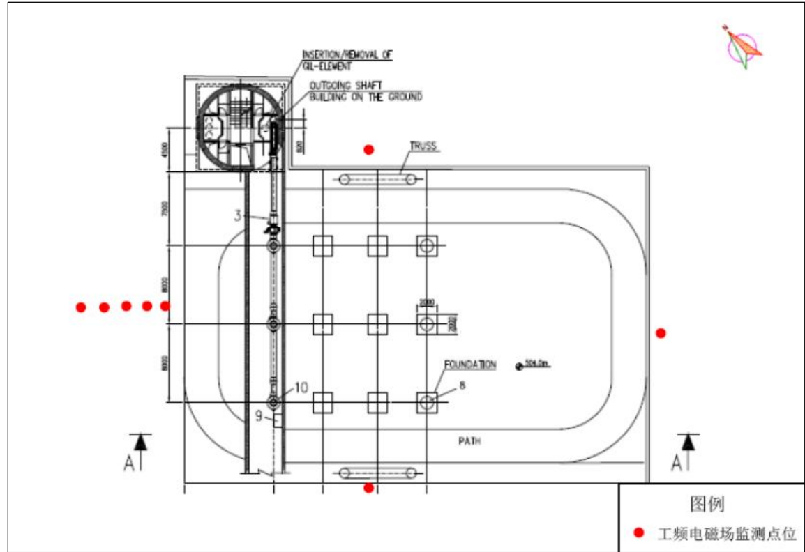
图 6.1-4 类比地面出线场工频电磁场监测点位
