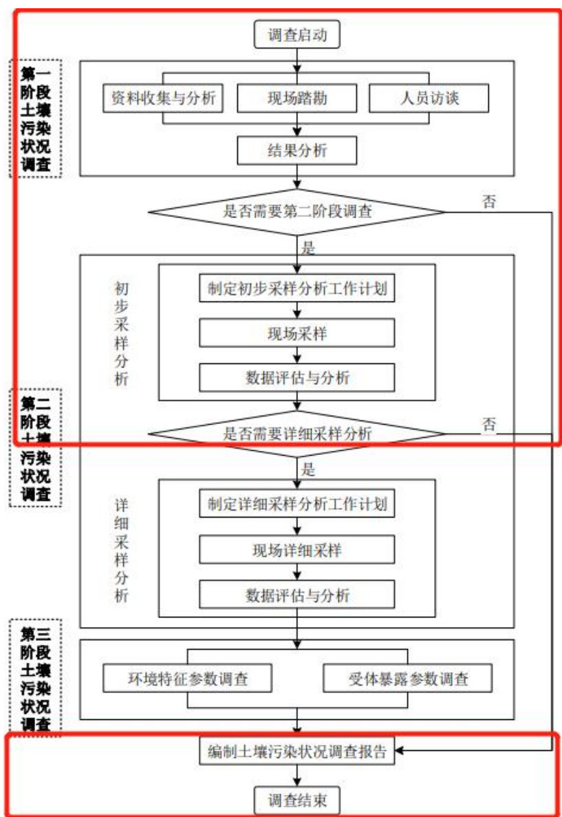
图 2-2 土壤污染状况调查的工作内容与程序
