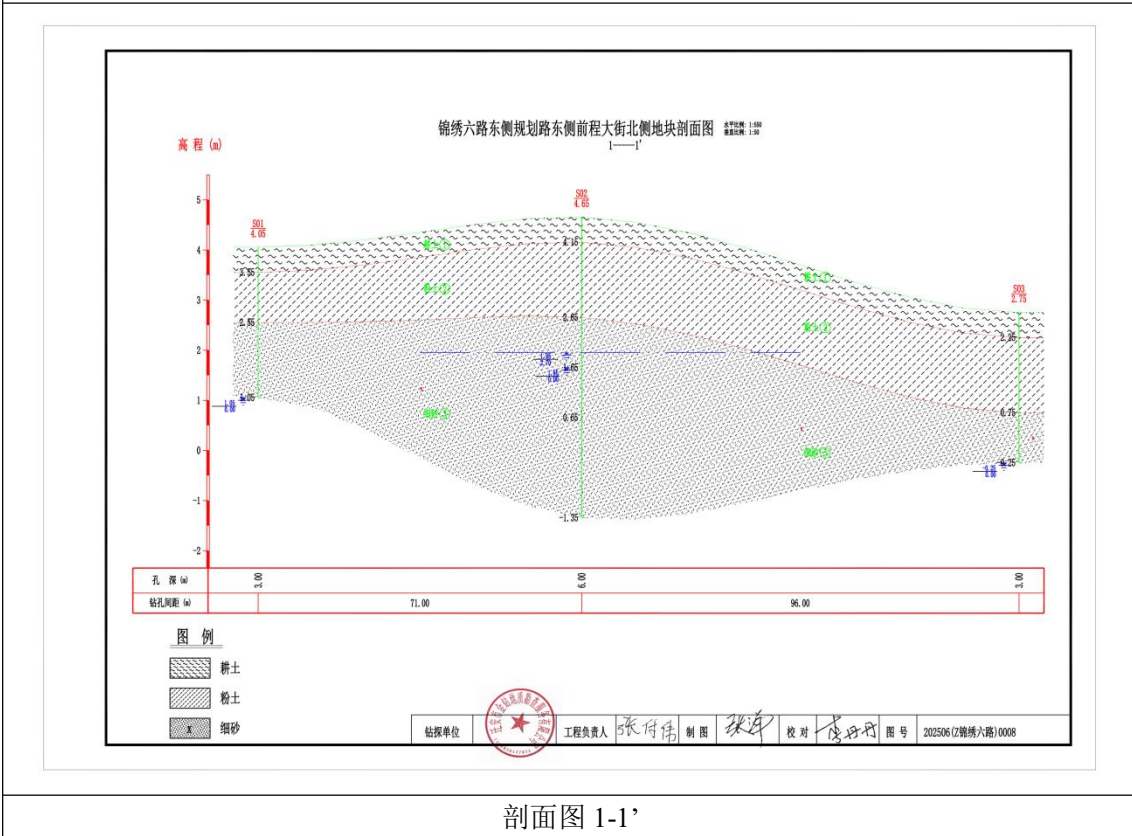
图 3-6 地块内钻孔剖面图
