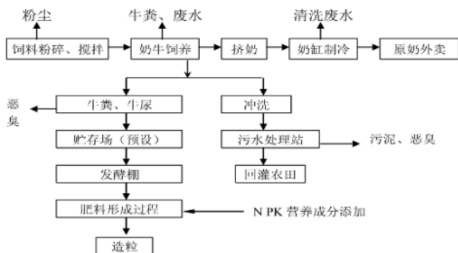
图 4.4-1 企业主要工艺流程图
