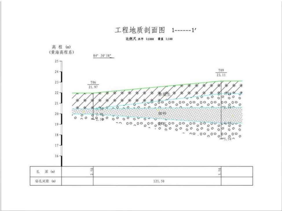
图 3-6 1-1' 线剖面图
