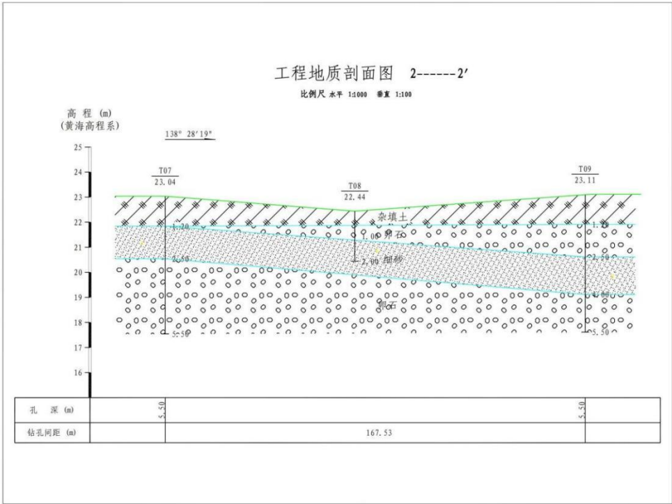
图 3-7 2-2' 线剖面图
