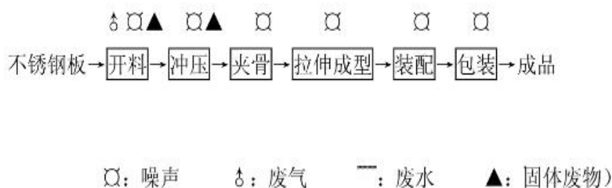
图 4.4-2 信拓金属主要工艺流程图
