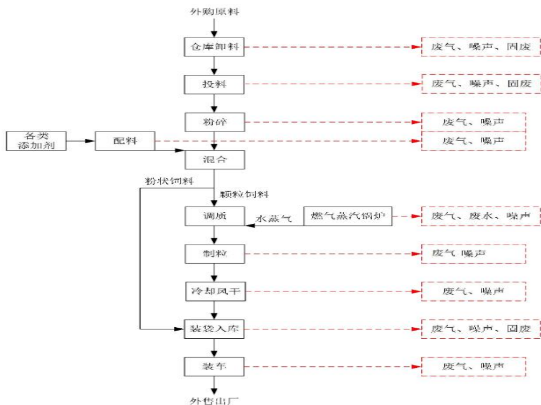
图 4.4-1 三富膨化饲料主要工艺流程图
